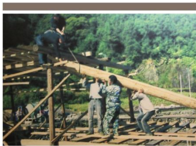
廊桥的建筑工艺流程：上三节苗
