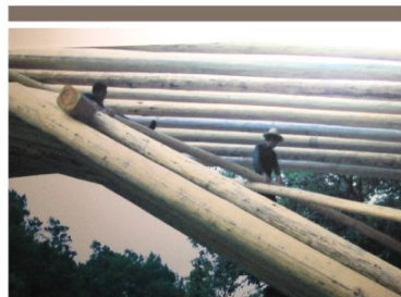
廊桥的建筑工艺流程：剪刀撑
